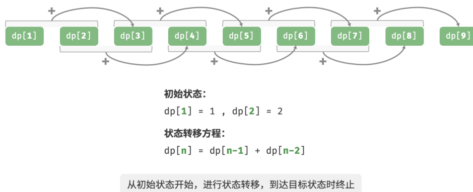
图 14-5 爬楼梯的动态规划过程
