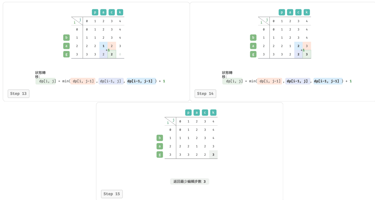
圖 14-30 編輯距離的動態規劃過程
