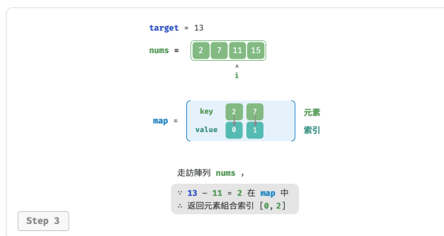
圖 10-10 輔助雜湊表求解兩數之和
