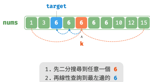
圖 10-5 線性查詢重複元素的插入點
