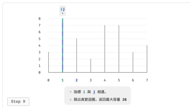
圖 15-11 最大容量問題的貪婪過程
