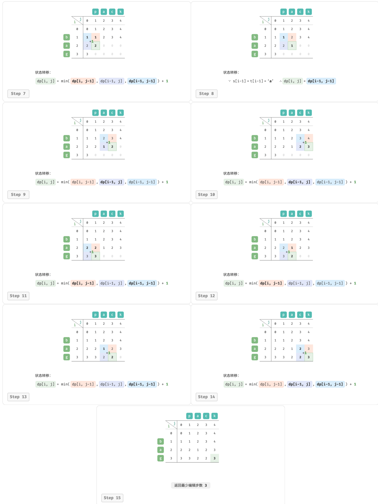
图 14-30 编辑距离的动态规划过程
