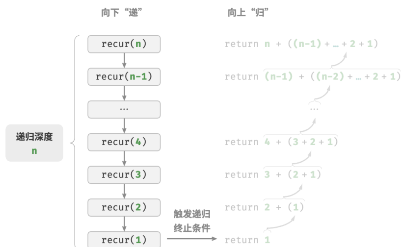
图 2-4 递归调用深度
