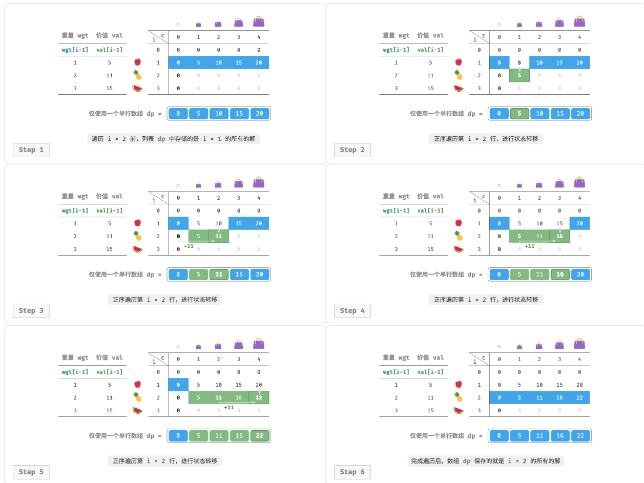
图 14-23 完全背包问题在空间优化后的动态规划过程
