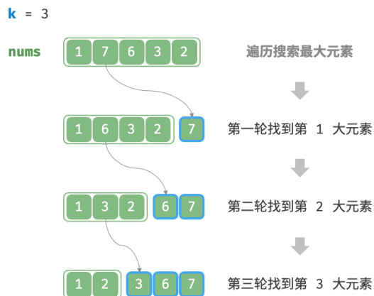
图 8-6 遍历寻找最大的 k 个元素
