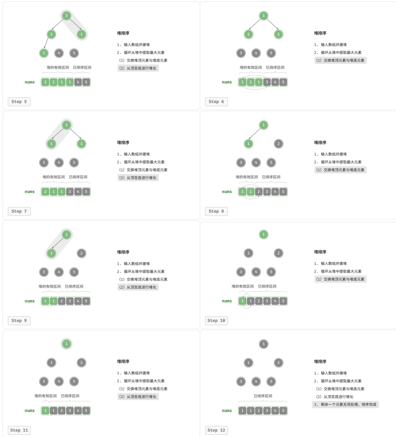
图 11-12 堆排序步骤
