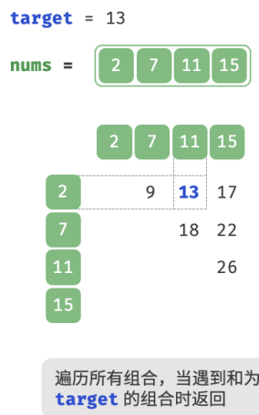
图 10-9 线性查找求解两数之和
