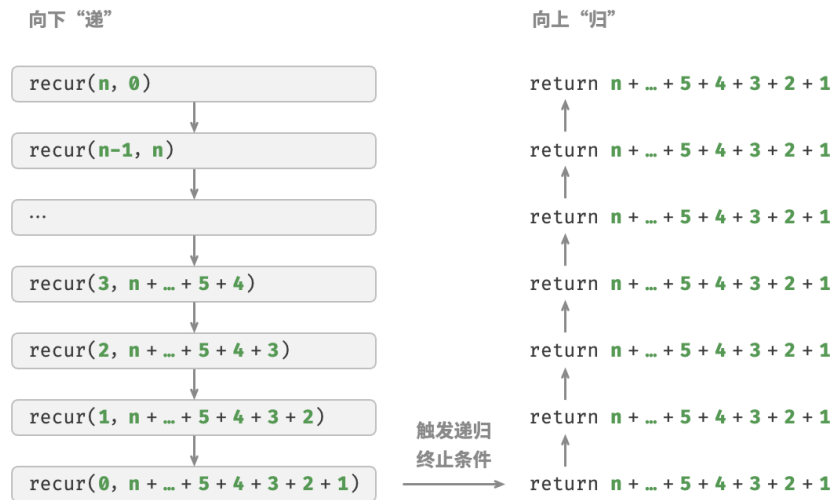
图 2-5 尾递归过程
