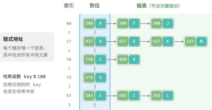
图 6-5 链式地址哈希表
