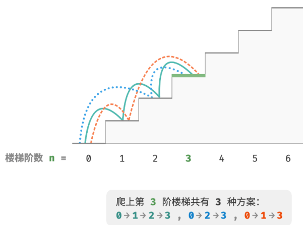
图 14-1 爬到第 3 阶的方案数量
