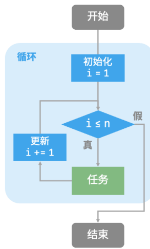
图 2-1 求和函数的流程框图
