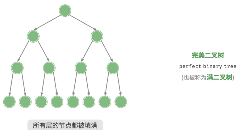
图 7-4 完美二叉树
