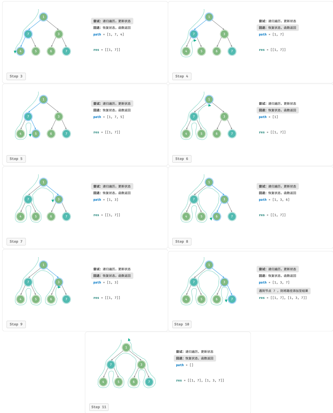
图 13-2 尝试与回退
