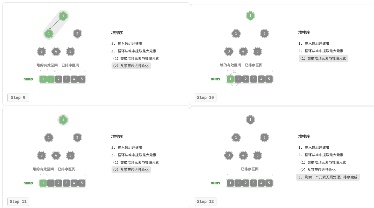
图 11-12 堆排序步骤
