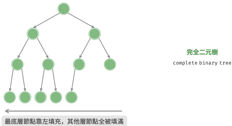
圖 7-5 完全二元樹
