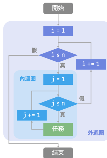
圖 2-2 巢狀迴圈的流程框圖
