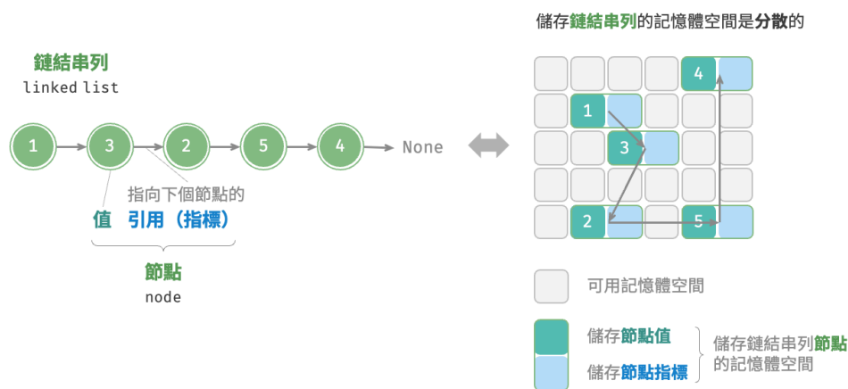
圖 4-5 鏈結串列定義與儲存方式
