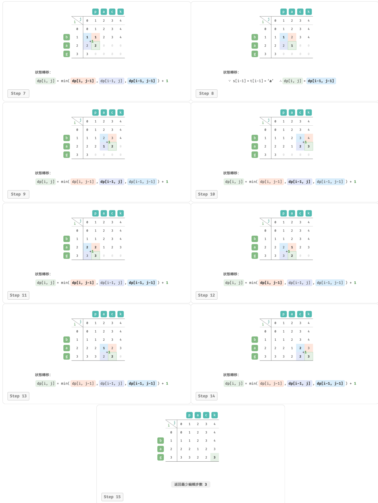
圖 14-30 編輯距離的動態規劃過程
