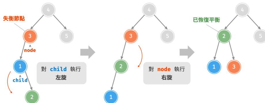
圖 7-30 先左旋後右旋
