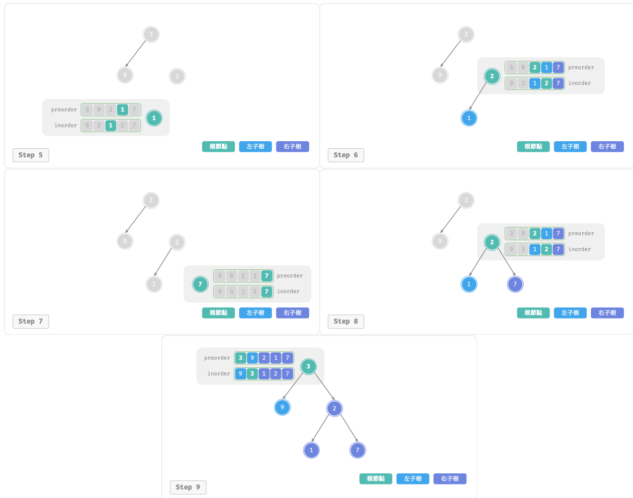
圖 12-8 構建二元樹的遞迴過程
