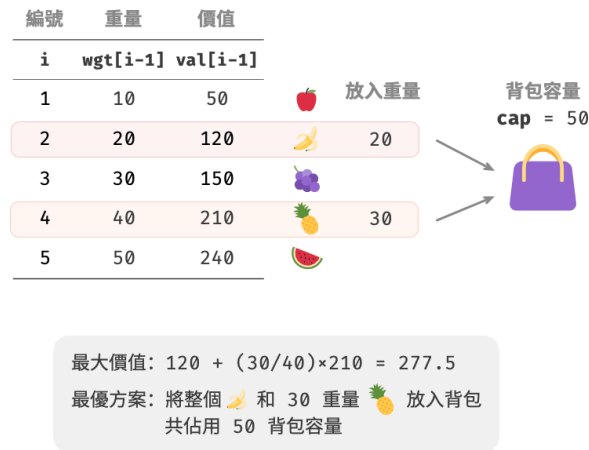
圖 15-3 分數背包問題的示例資料
