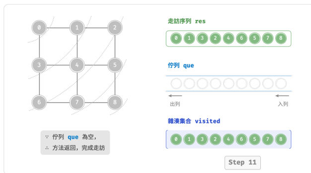
圖 9-10 圖的廣度優先走訪步驟
