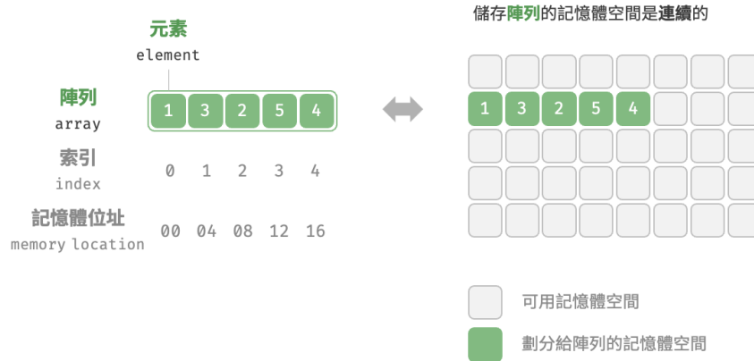
圖 4-1 陣列定義與儲存方式
