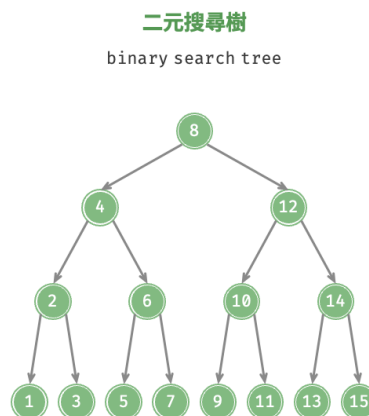
圖 7-16 二元搜尋樹
