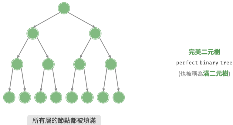
圖 7-4 完美二元樹
