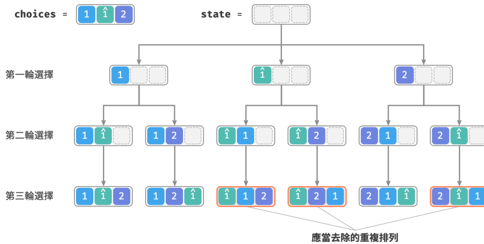
圖 13-7 重複排列
