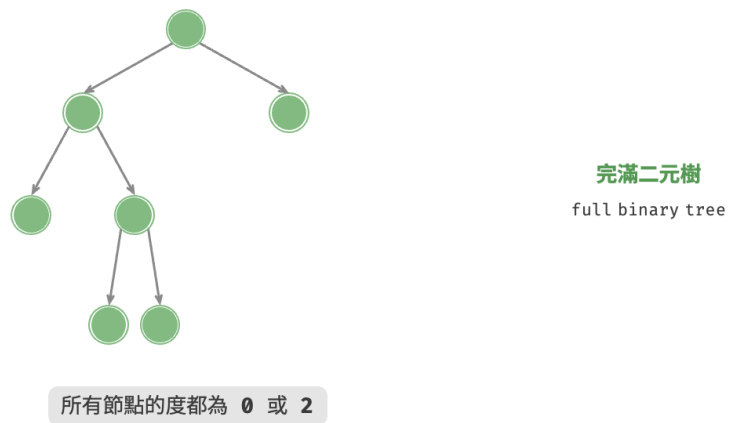
圖 7-6 完滿二元樹
