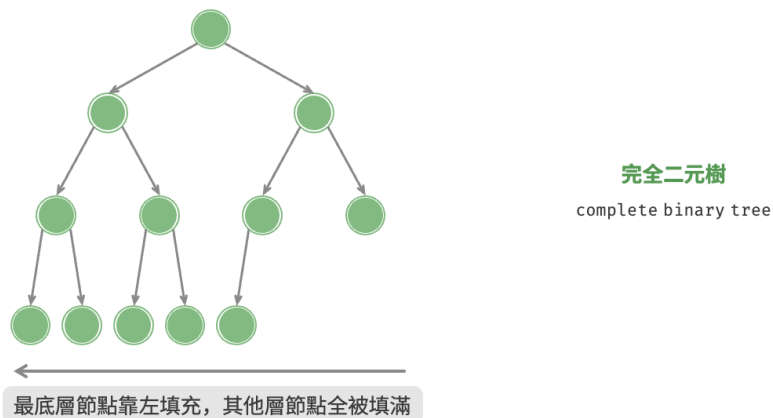
圖 7-5 完全二元樹
