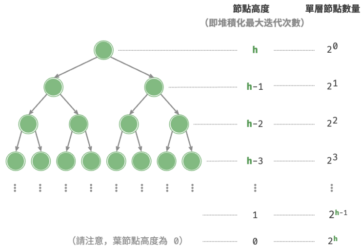
圖 8-5 完美二元樹的各層節點數量
