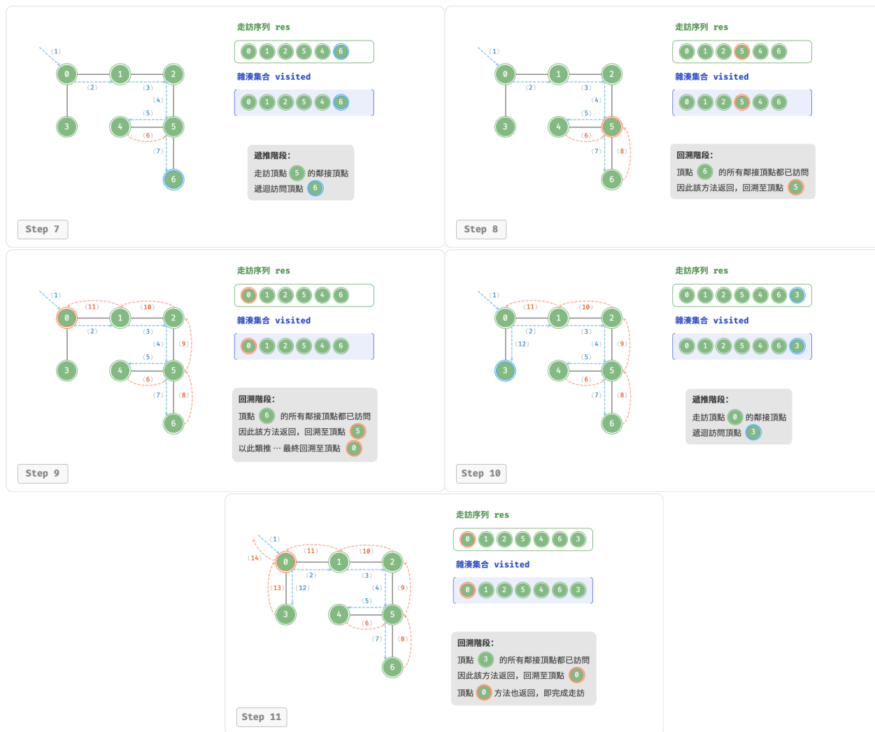
圖 9-12 圖的深度優先走訪步驟
