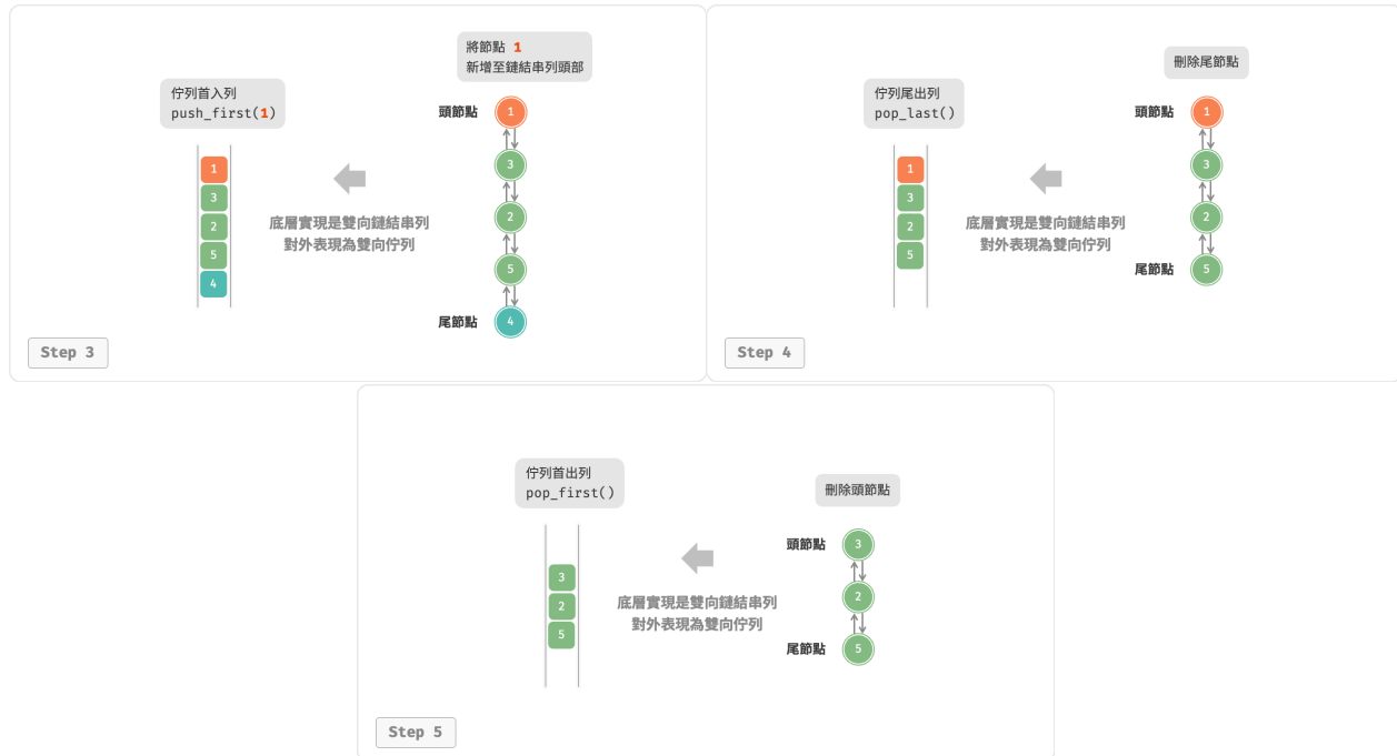
圖 5-8 基於鏈結串列表實現雙向佇列的入列出列操作
