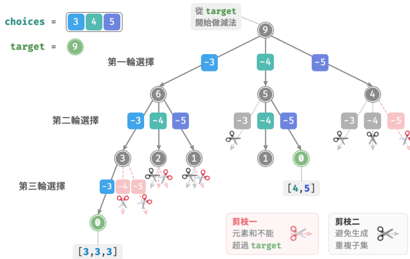
圖 13-12 所示為將陣列 [3, 4, 5] 和目標元素 9 輸入以上程式碼後的整體回溯過程。
