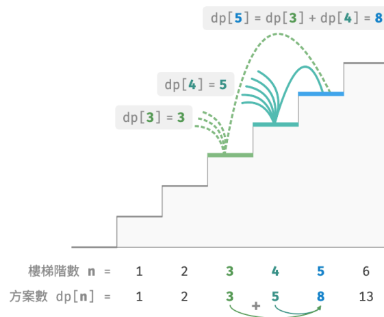
圖 14-2 方案數量遞推關係
