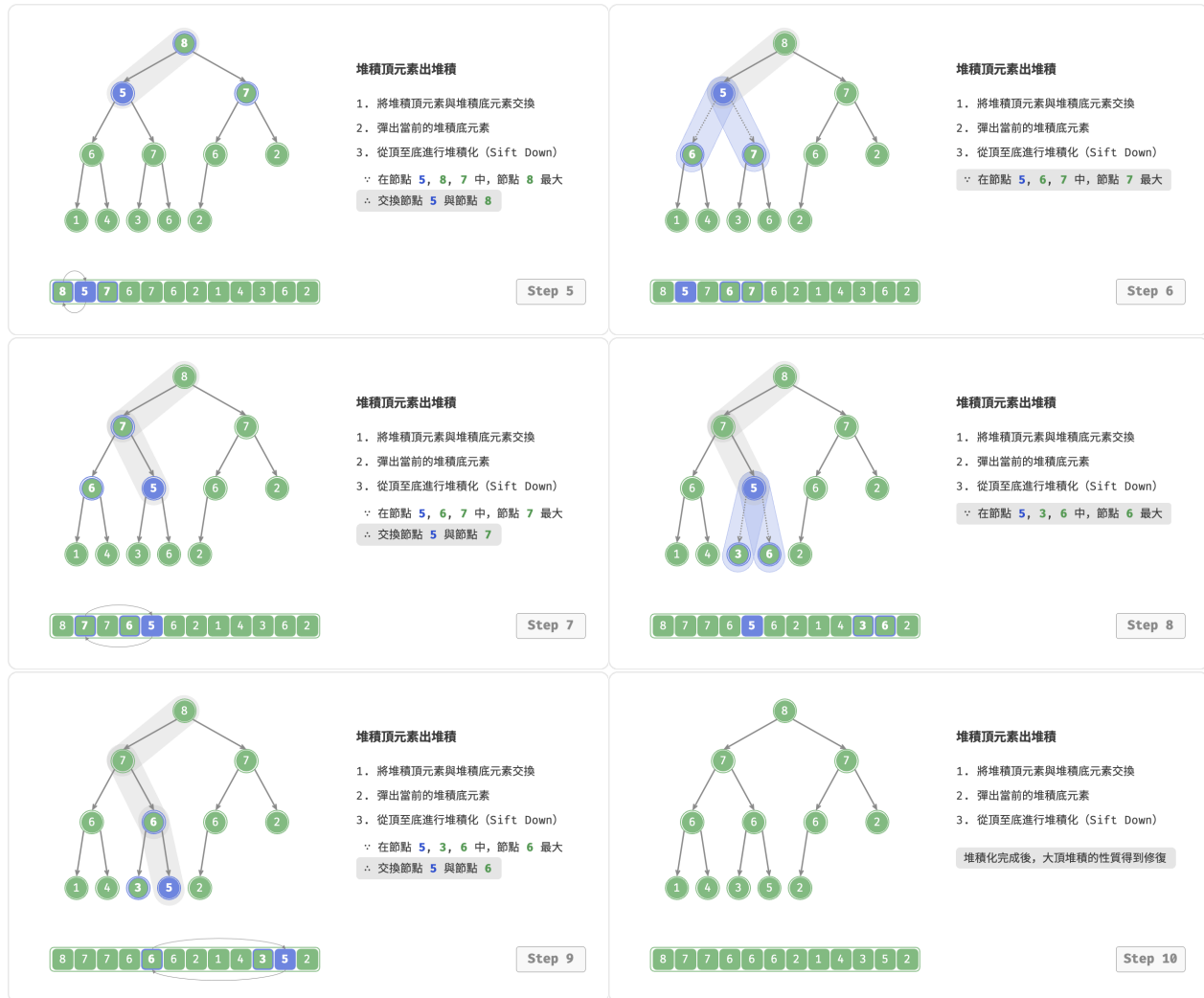
圖 8-4 堆積頂元素出堆積步驟
