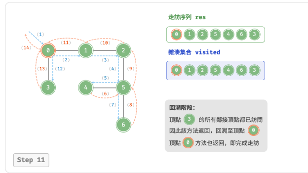
圖 9-12 圖的深度優先走訪步驟
