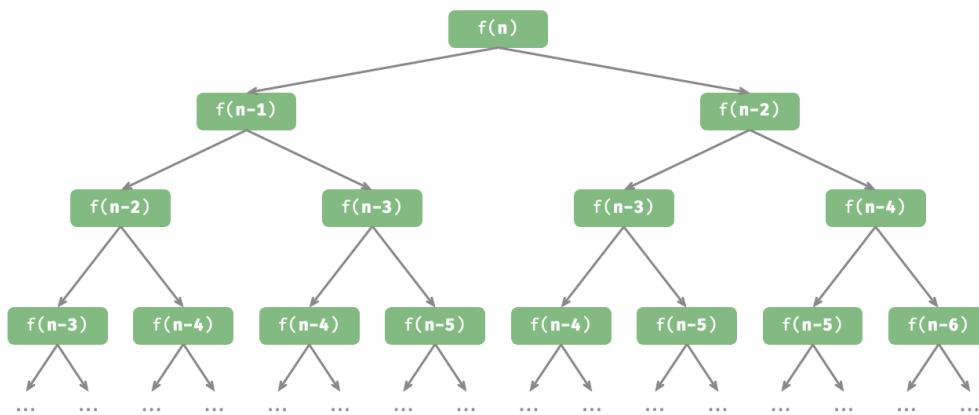
圖 2-6 費波那契數列的遞迴樹
