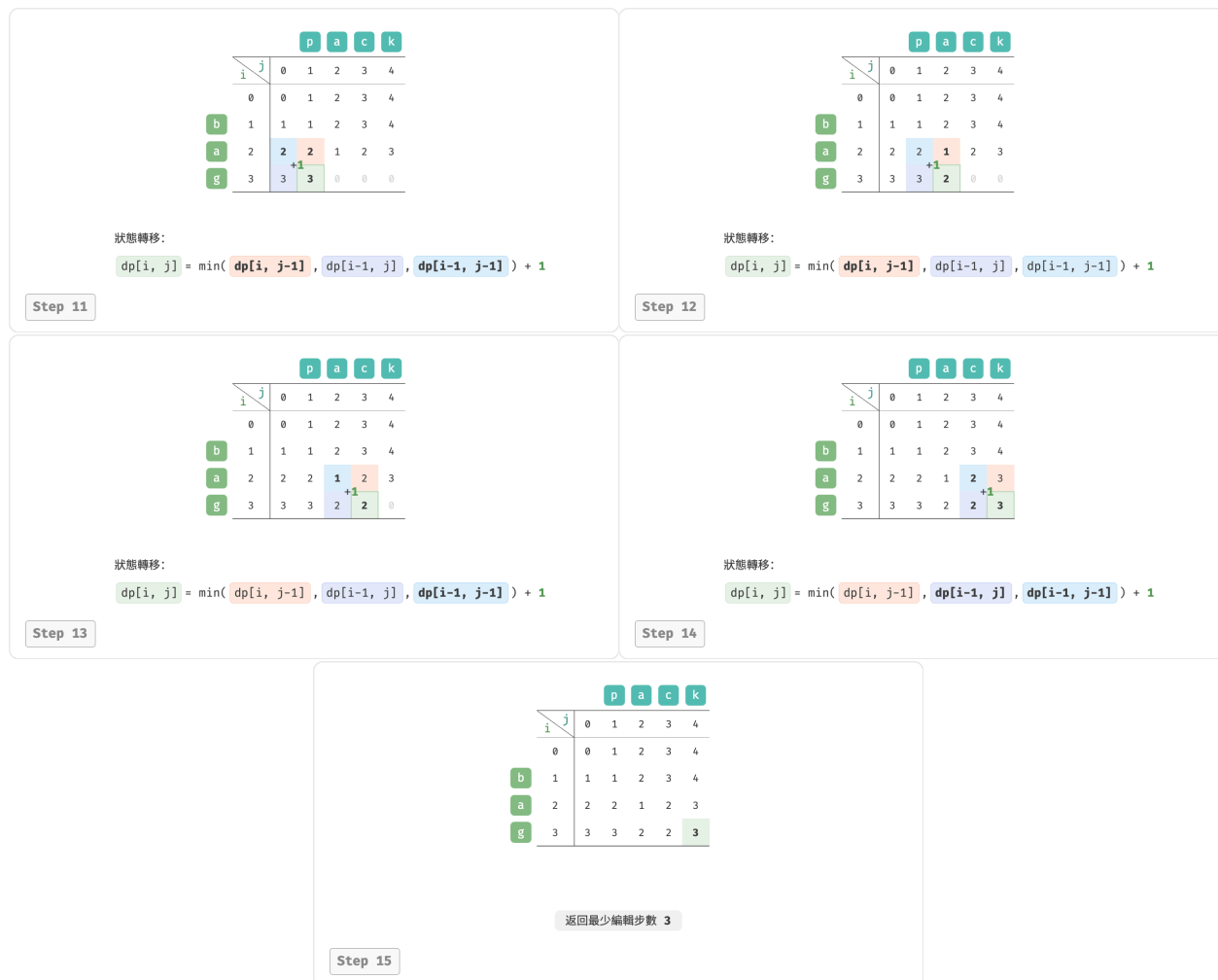
圖 14-30 編輯距離的動態規劃過程
