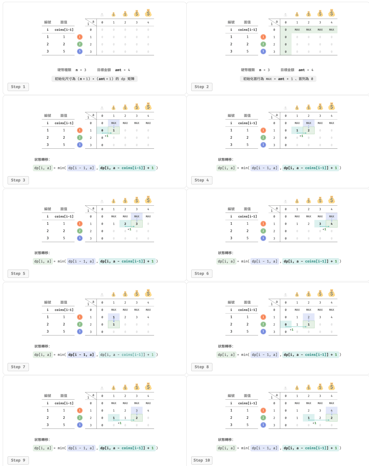
圖 14-25 展示了零錢兌換的動態規劃過程，和完全背包問題非常相似。
