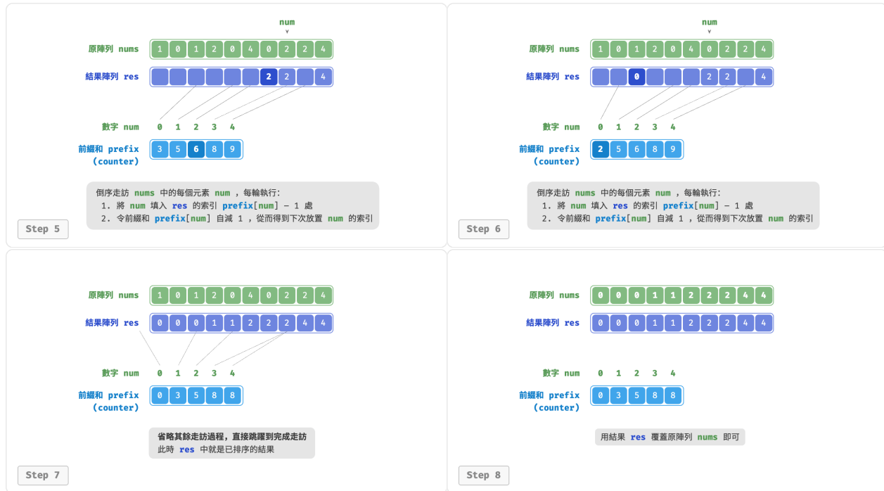
圖 11-17 計數排序步驟
