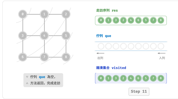
圖 9-10 圖的廣度優先走訪步驟
