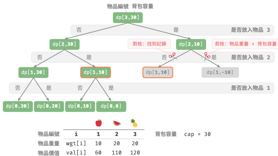
圖 14-19 展示了在記憶化搜尋中被剪掉的搜尋分支。
