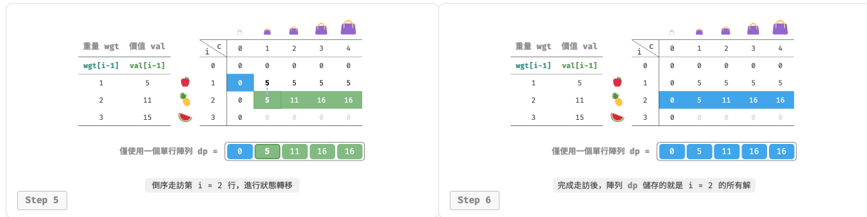
圖 14-21 0-1 背包的空間最佳化後的動態規劃過程
