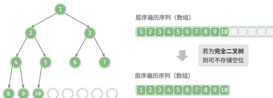
图 7-15 完全二叉树的数组表示
