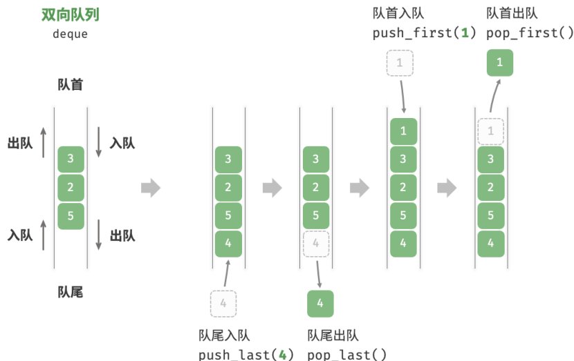
图 5-7 双向队列的操作
