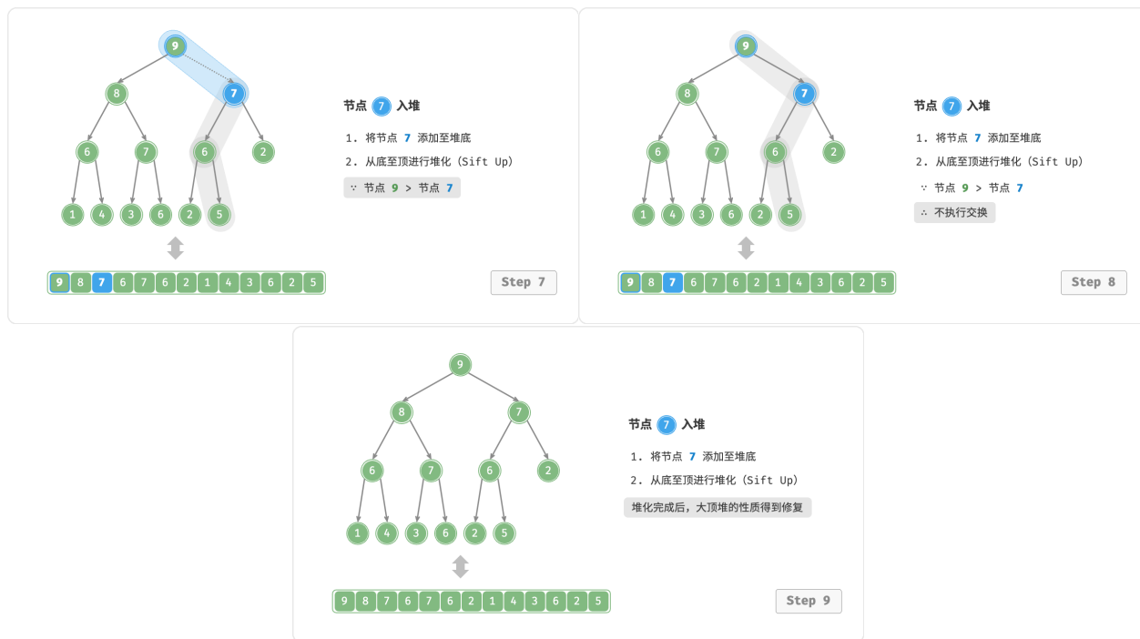
图 8-3 元素入堆步骤
