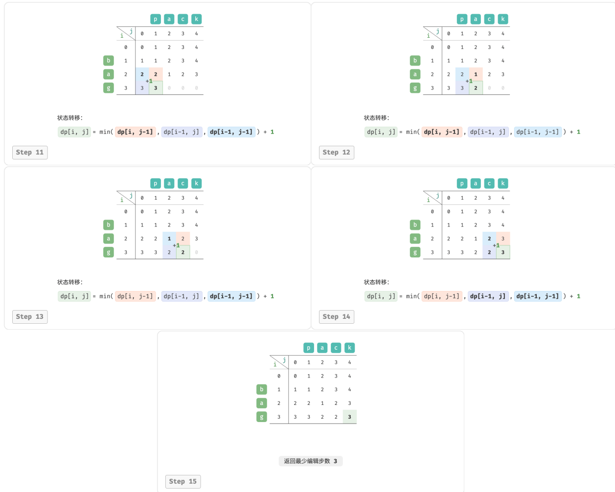
图 14-30 编辑距离的动态规划过程
