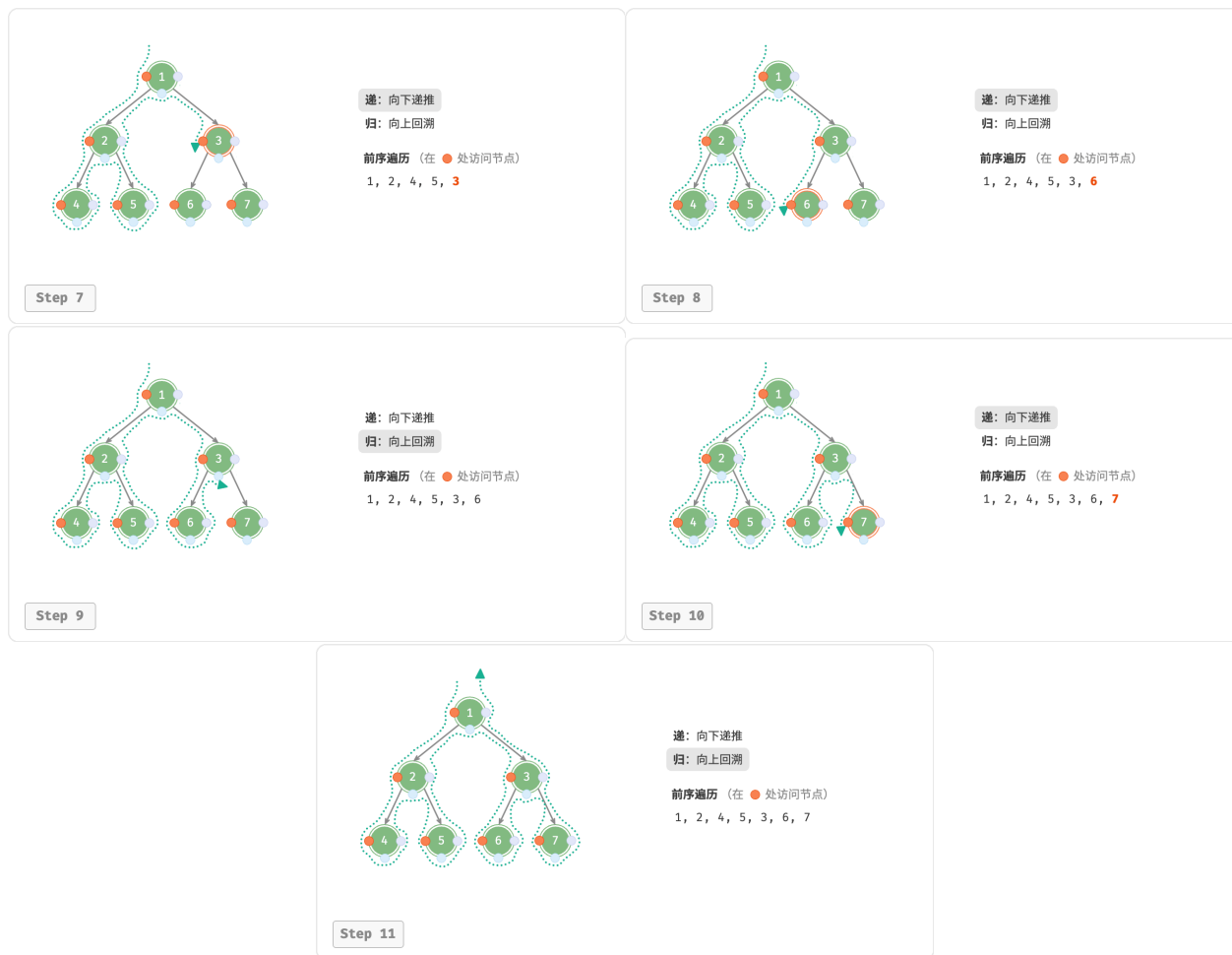
图 7-11 前序遍历的递归过程
