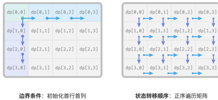
图 14-13 边界条件与状态转移顺序
