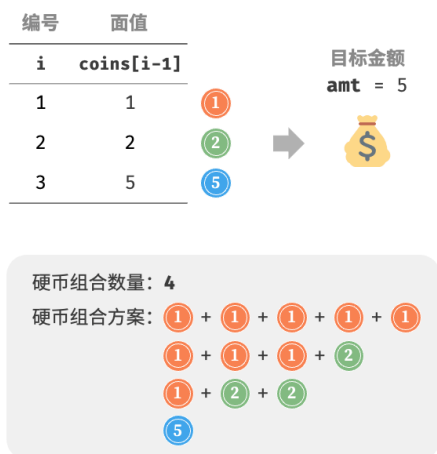
图 14-26 零钱兑换问题 II 的示例数据
