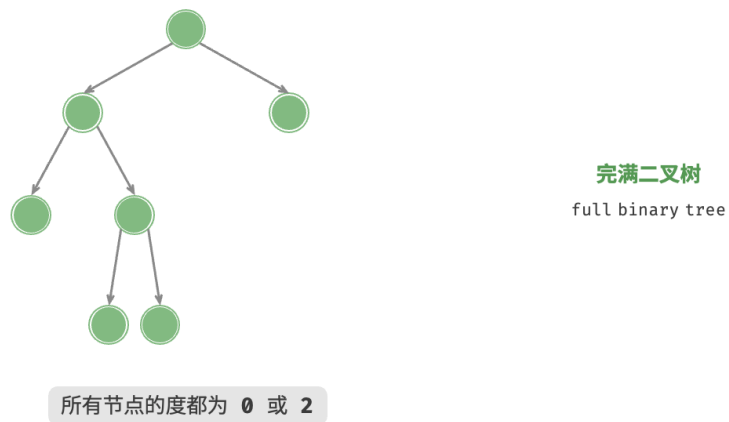
图 7-6 完满二叉树
