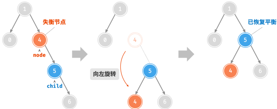
图 7-28 左旋操作
