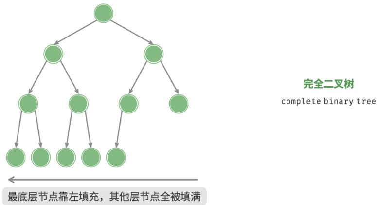
图 7-5 完全二叉树
